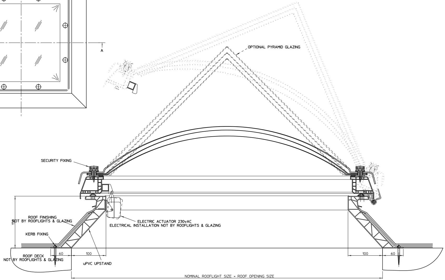
SECTION A-A
