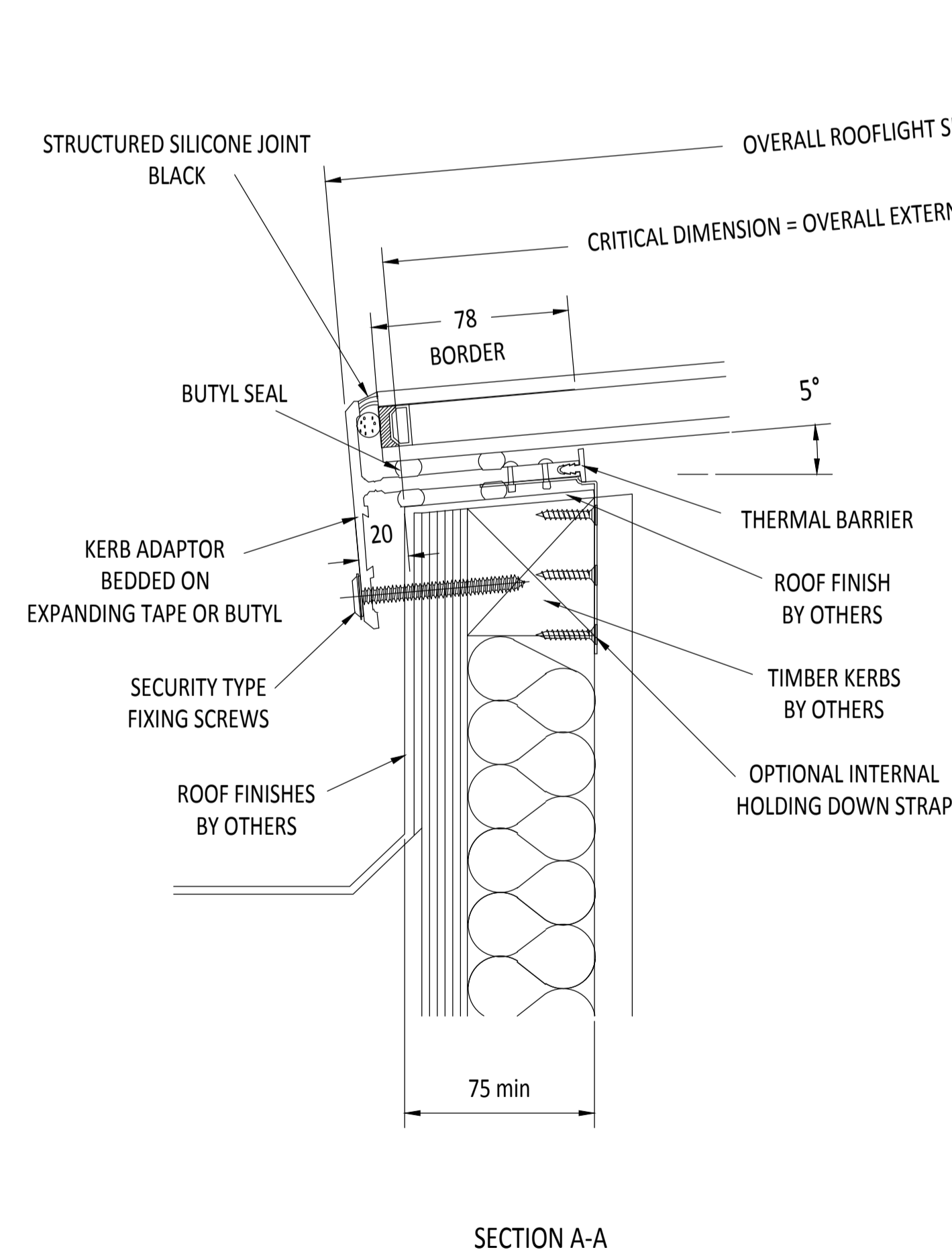
SECTION A-A
